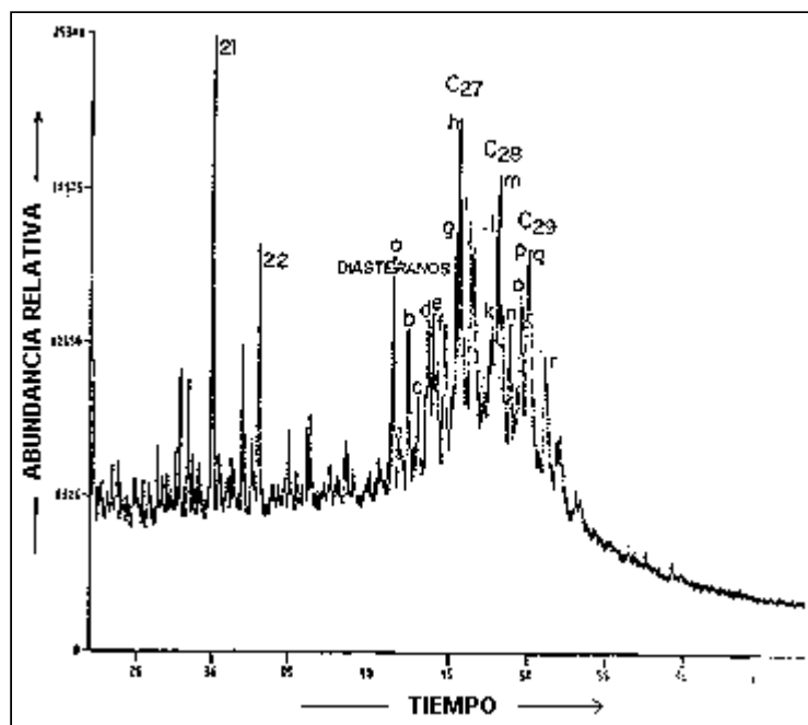
Distribución de biomarcadores esteranos m/z 217 del mene Mene Grande (Tomado de: Del Olio, 1993)
