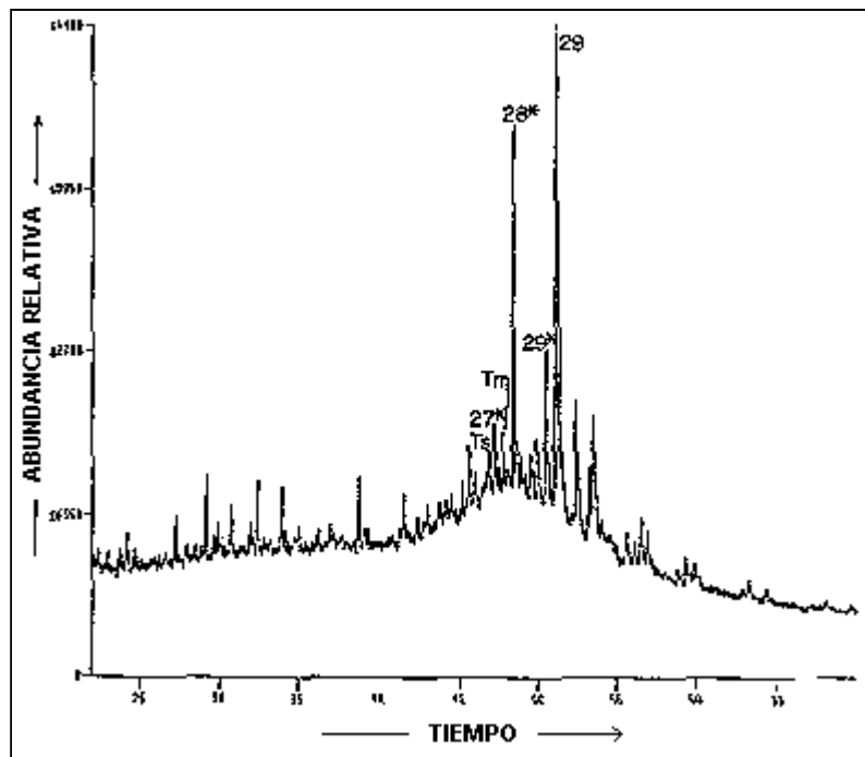
Distribución de biomarcadores terpanos m/z 191(a) y m/z 177(b) del mene de Mene Grande (Tomado de: Del Olio, 1993)
