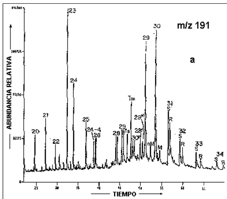
Cromatograma de la fracción saturada del mene de Mene Grande (Tomado de: Del Olio, 1993)
