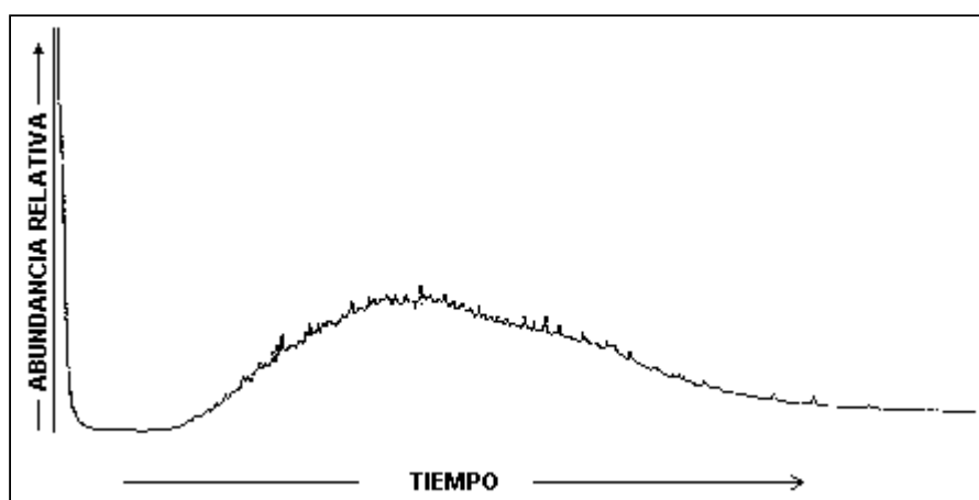
Cromatograma de la fracción saturada del mene de Mene Grande (Tomado de: Del Olio, 1993)
